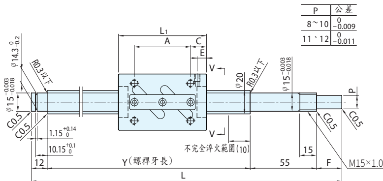
螺桿軸徑20
