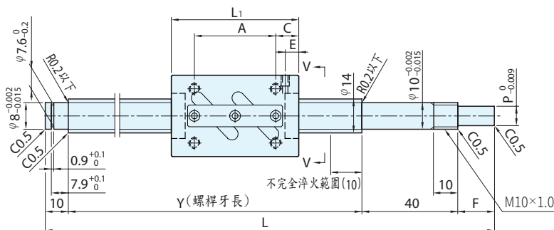
螺桿軸徑14
