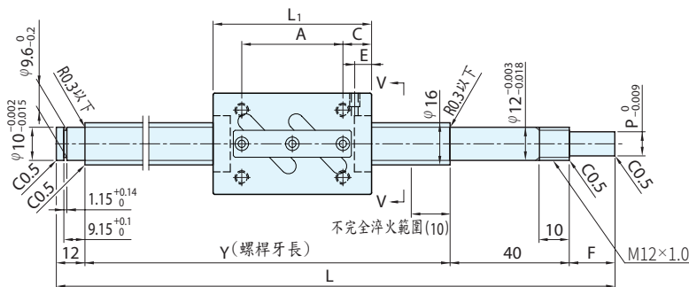
螺桿軸徑16
